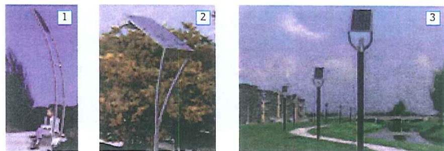
Fig.1 - Modelli studio, Ecofys Fig.2 - Modello Bambù, fonte Ecofys Fig.3 - Modello Ecolux3, fonte Ecofys
